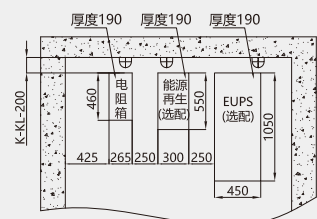
E向
