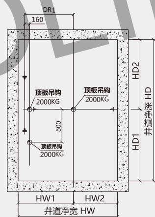
井道平面吊钩图 (吊钩用户自理)
