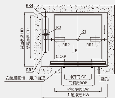
井道平面图
