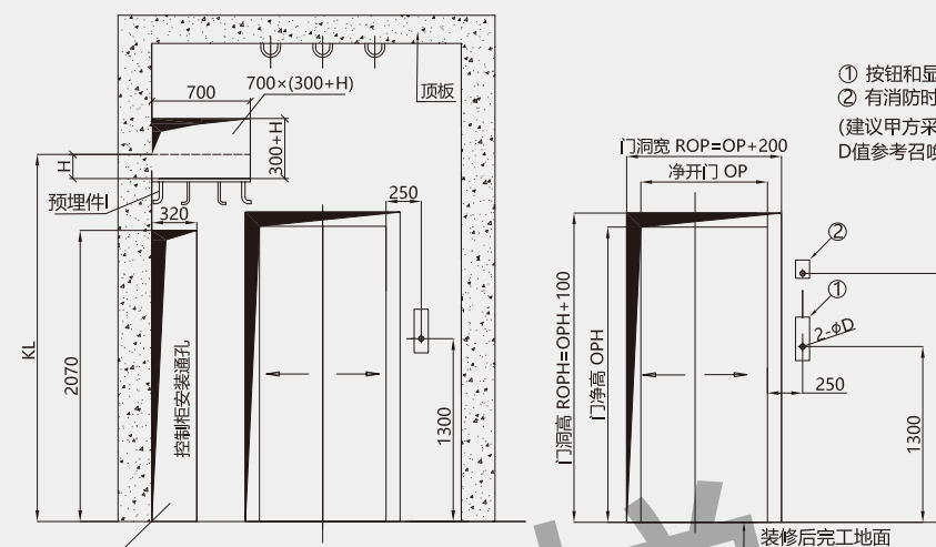
顶层厅门图
