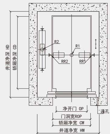
井道平面图
